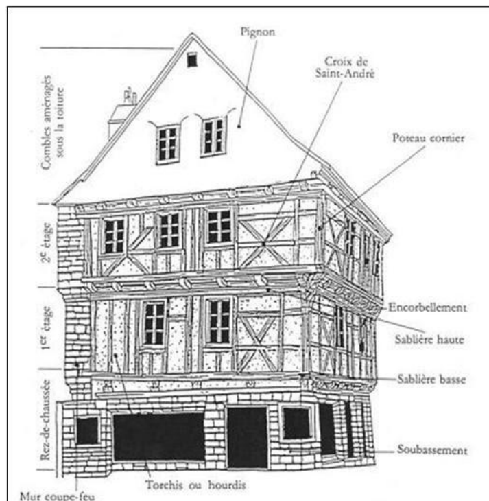
Schéma descriptif d'une maison à pan de bois
